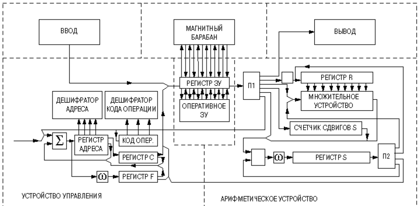
Блок-схема вычислительной машины "Сетунь"
